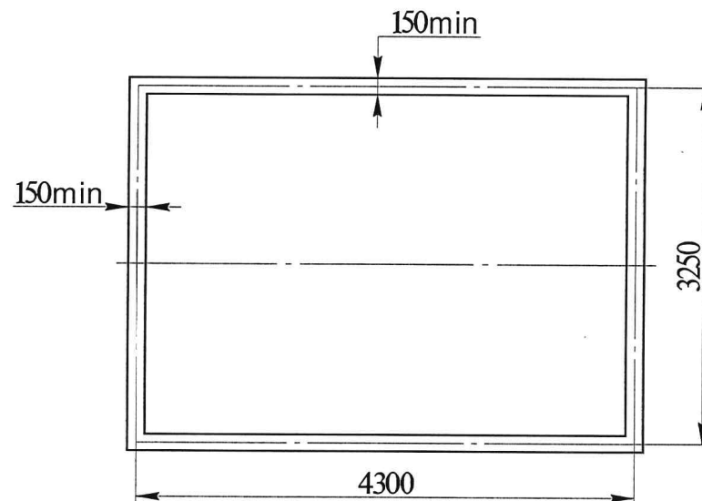
План фундамента
