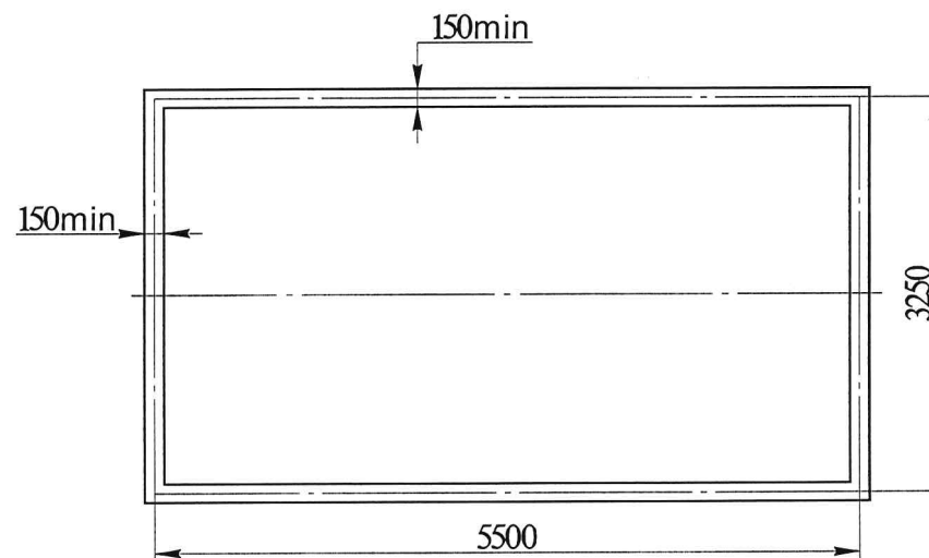
План фундамента
