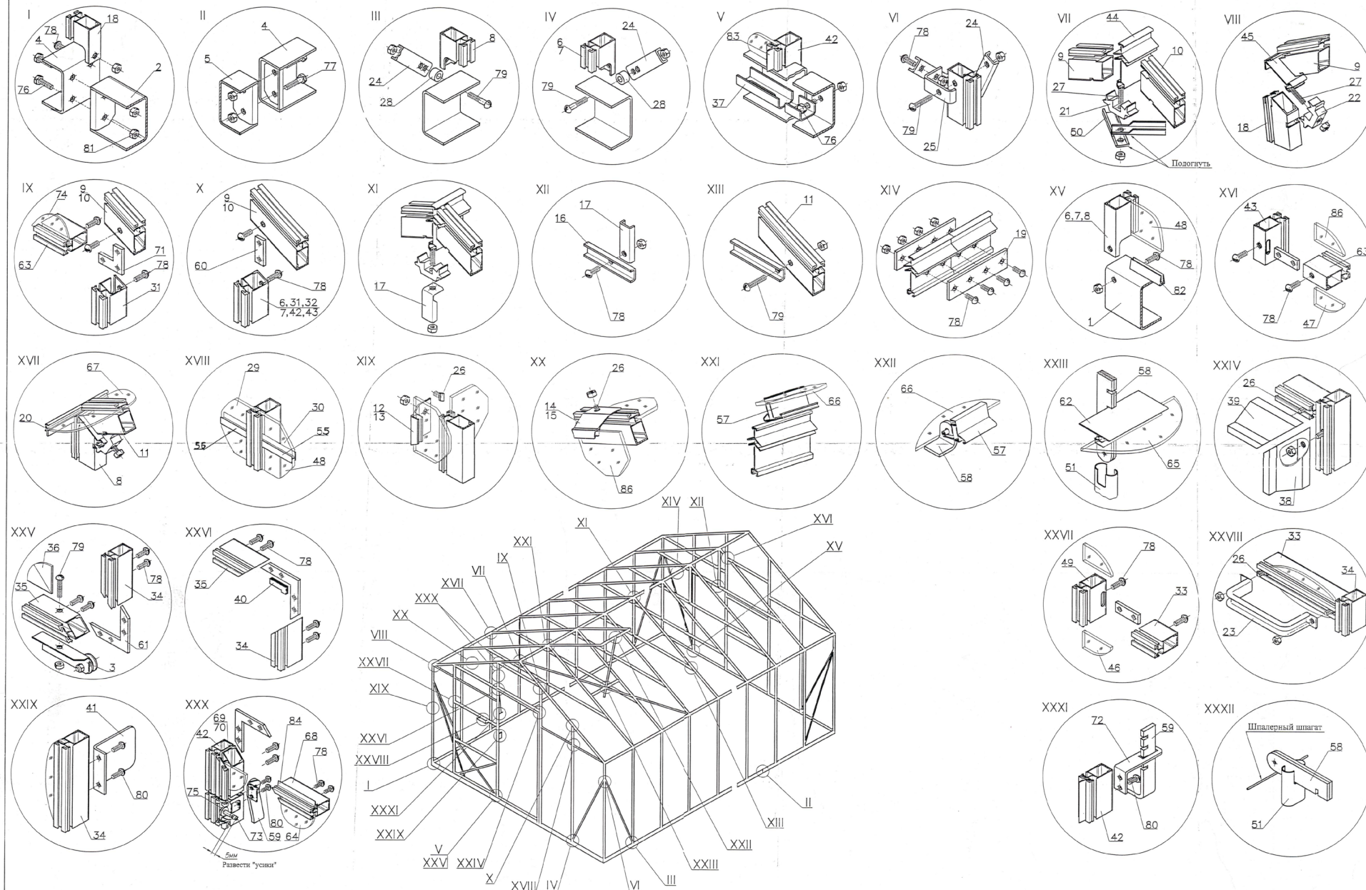
Рисунок. Схема сборки теплицы
