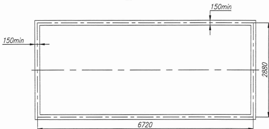
План фундамента
