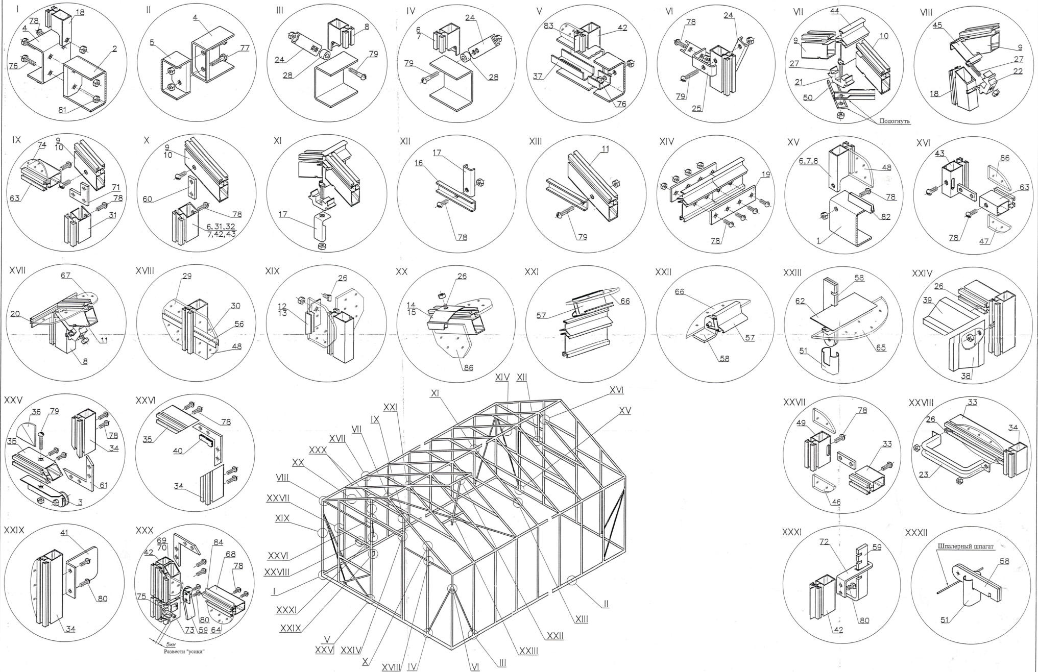
Рисунок. Схема сборки теплицы Торцевая форточка с элементами крепления и фиксации условно показана на торце с дверью
